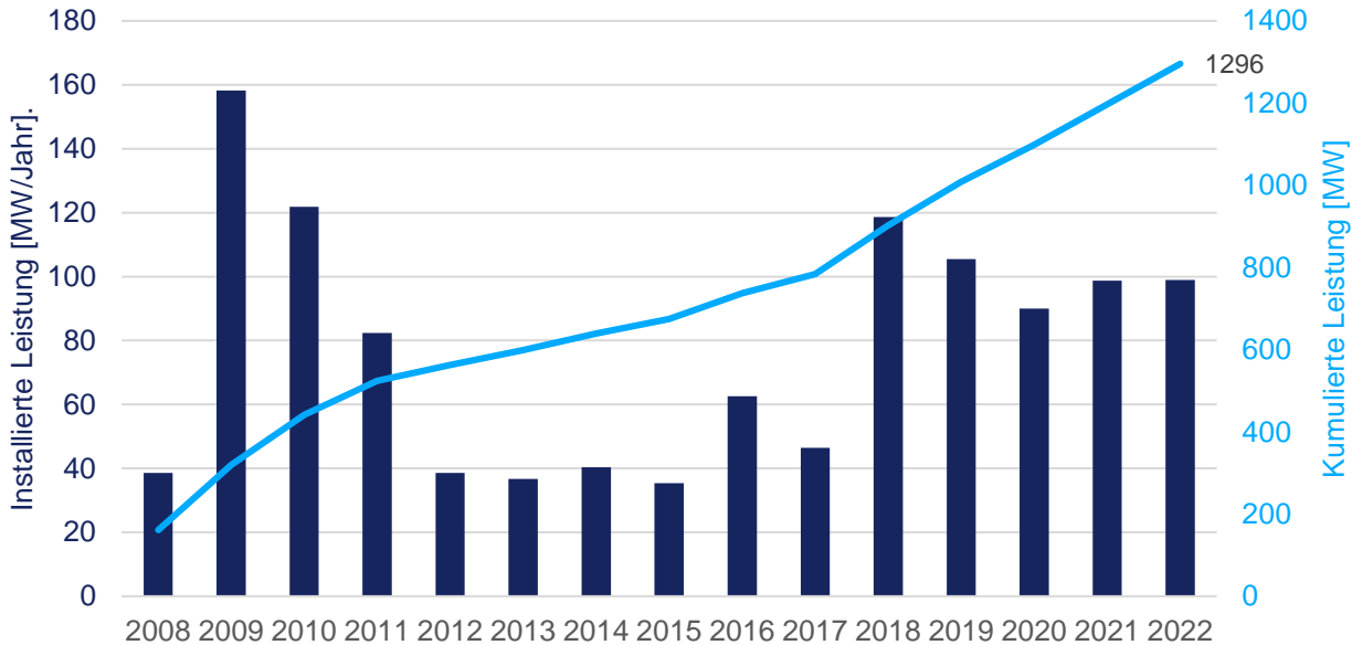
Entwicklung der installierten Kapazitäten
